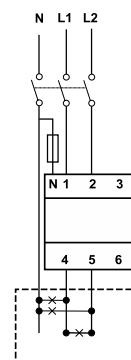
Fig. 7 Biphasé (3 fils)
